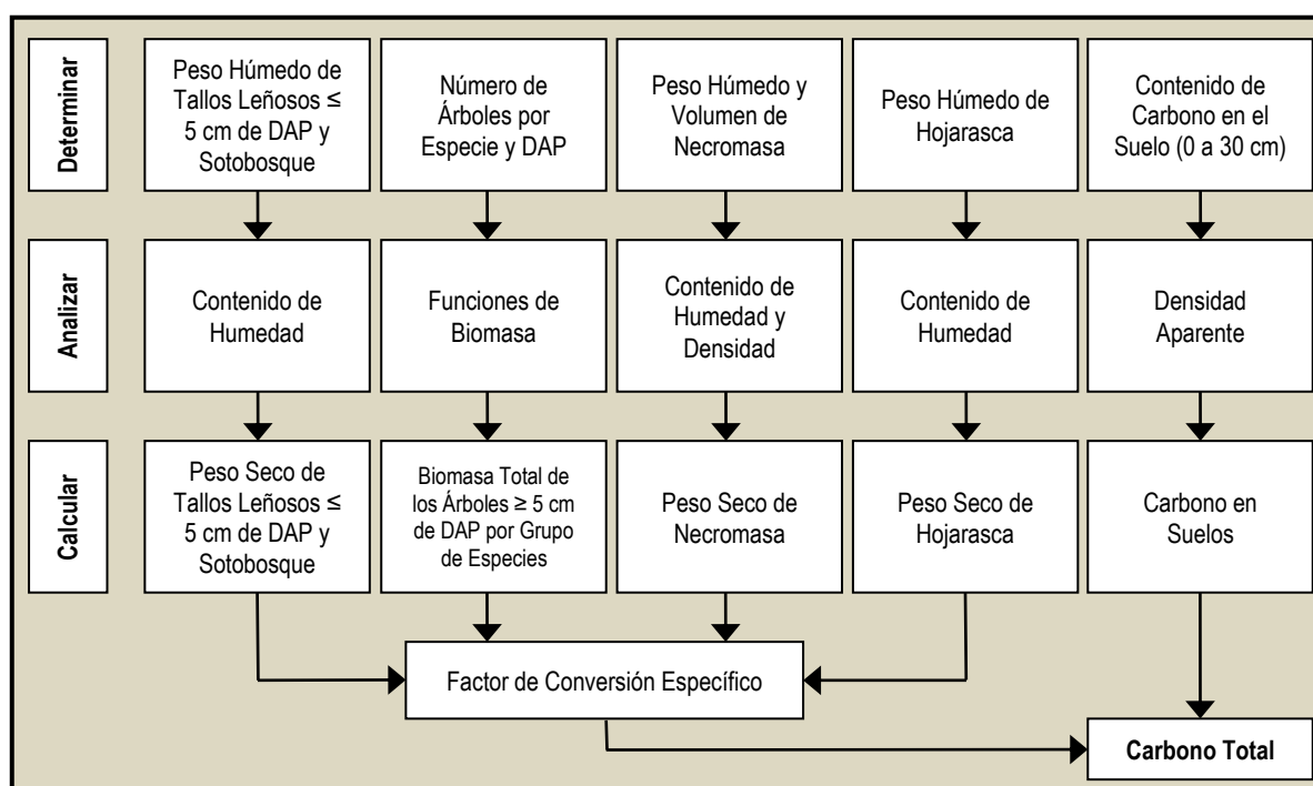
Figura 15. Diagrama de flujo para calcular el carbono en los principales depósitos en ecosistemas forestales.
