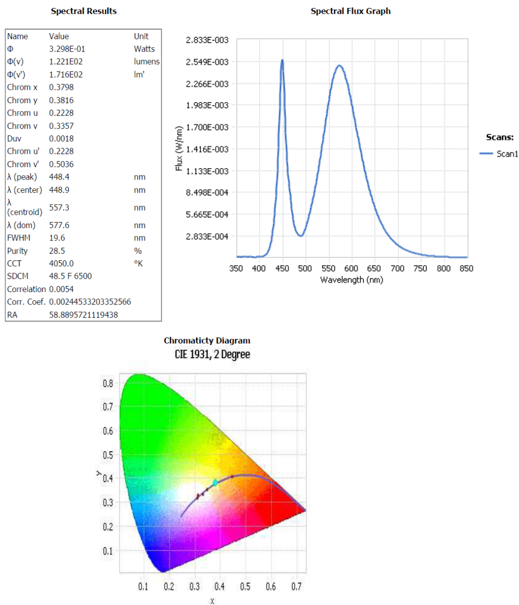
Figura 56: Resultados de la lámpara Sun King Pro realizada por la esfera LMS-400.
