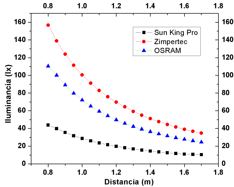
Figura 36: Iluminancia versus la distancia.
