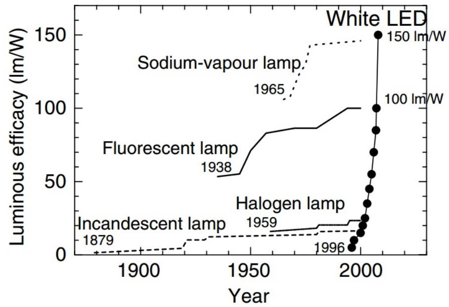
Figura 1: Historia de la eficacia de diferentes lámparas [2].
