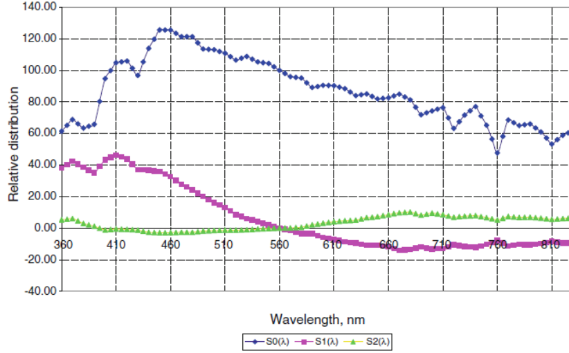
Figura 8: Funciones características para poder construir las fases del día[15].
