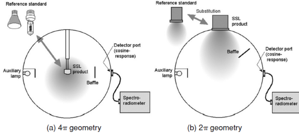
Figura 15: Geometrías 2\pi y 4\pi para el uso de una esfera integradora con un espectralradiómetro [32].
