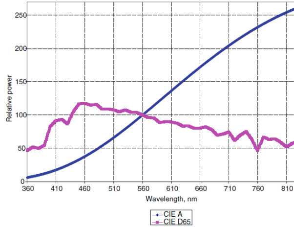
Figura 7: La linea azul representa la iluminante CIE A y la linea morada representa la iluminante CIE D65 [15].
