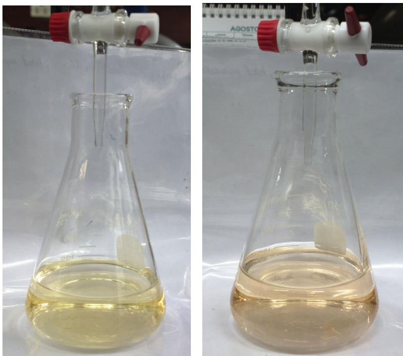
Figura 21. Determinación de alcalinidad total. Punto inicial de titulación (izquierda) y punto final de titulación (derecha). Fuente: Propia
