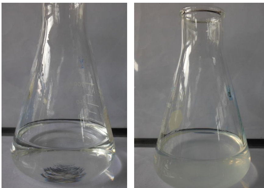
Figura 24. Determinación de sulfatos. Muestra antes de agregar el \text{BaCl}_2 (izquierda) y después de agregar la sal (derecha). Fuente: Propia
